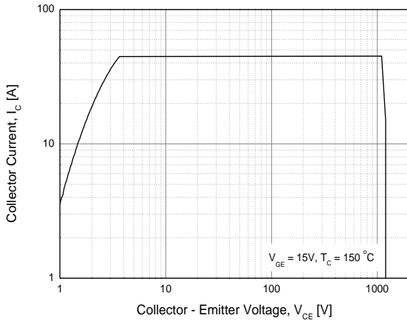
Fig. 15 RBSOA
