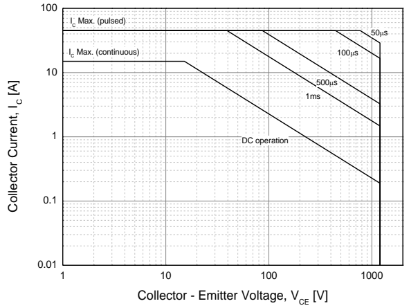
Fig. 14 SOA
